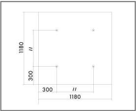
Схема установки пружинных анкеров для панели 1180 x 1180
