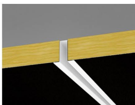
Фрагмент системы Акусто NE на стены с U-профилем
