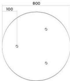
Схема установки пружинных анкеров для панели ø 800
