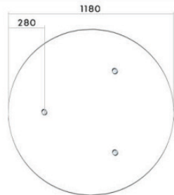
Схема установки пружинных анкеров для панели ø 1180
